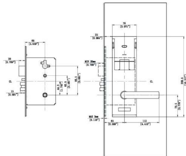
EURO lockcase
