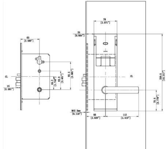
AUS lockcase
