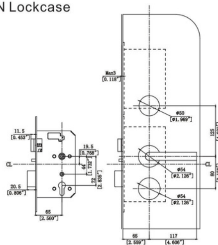
DIN Lockcase
