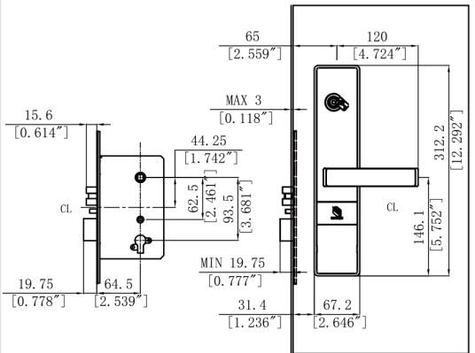
EURO Lockcase
