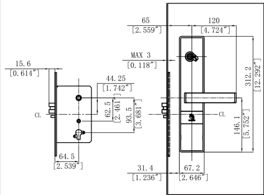
AUS Lockcase
